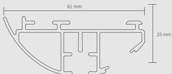
Gemotoriseerd DS-XL LED Kleuren: wit & antraciet
