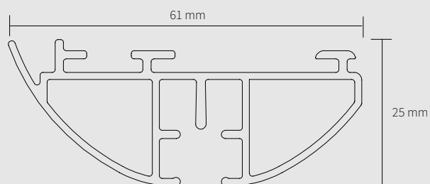
Gemotoriseerd DS-XL Kleuren: mat wit & mat zwart
